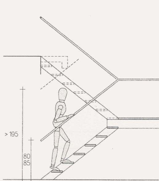
escadas residenciais 25-45gr
