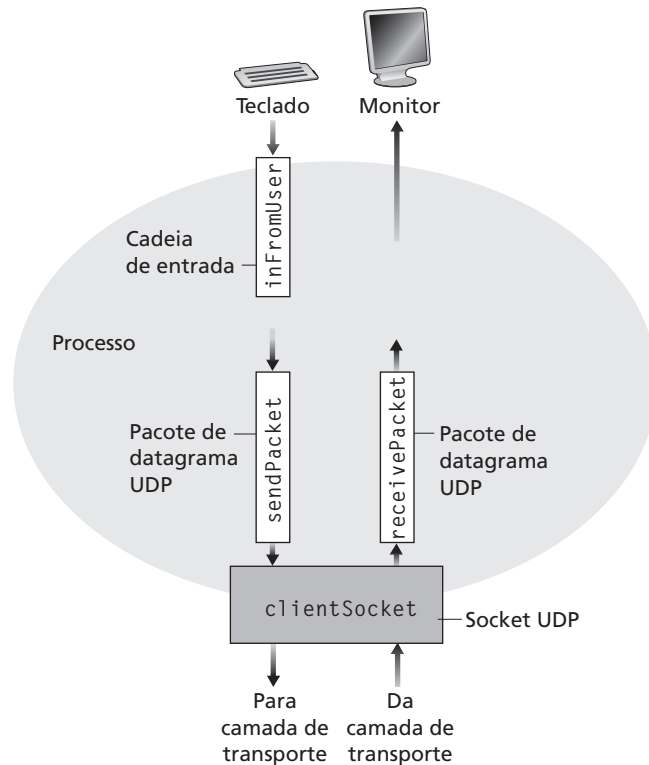
Figura 2.33 UDPClient tem uma corrente; o socket aceita pacotes do processo e entrega pacotes ao processo
