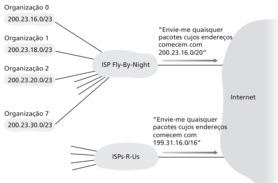
Figura 4.18 Endereçamento hierárquico e agregação de rotas
