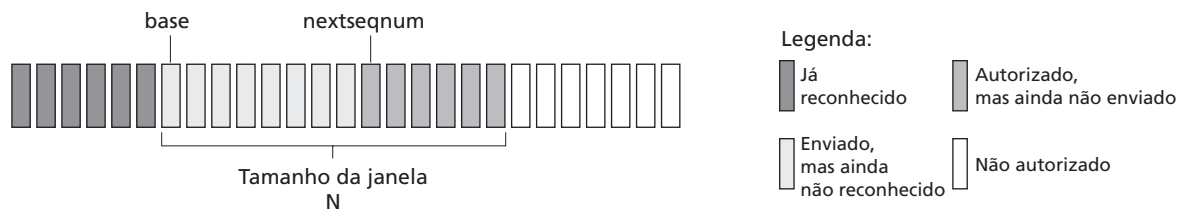
Figura 3.19 Visão do remetente para os números de sequência no protocolo Go-Back-N
