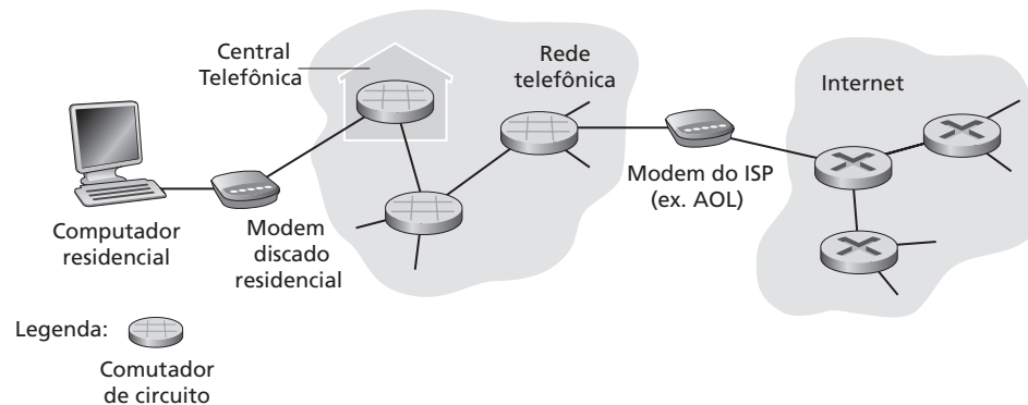
Figura 1.5 Acesso à Internet discado
