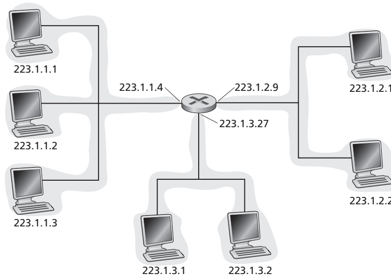
Figura 4.15 Endereços de interfaces e sub-redes
