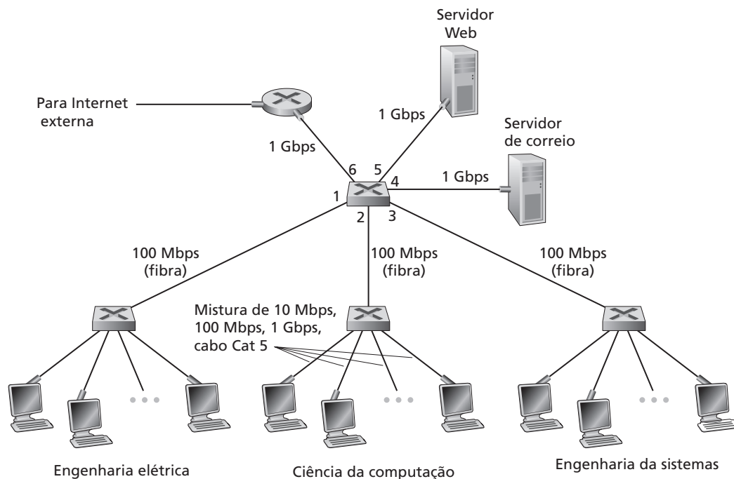
Figura 5.26 Três Ethernets departamentais interconectados com um hub
