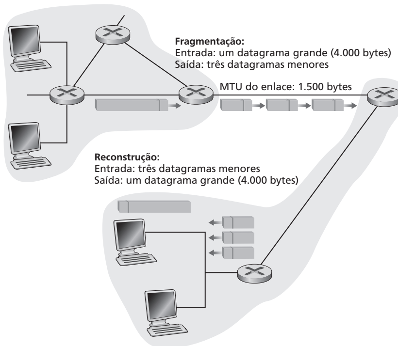
Figura 4.14 Fragmentação e reconstrução IP
