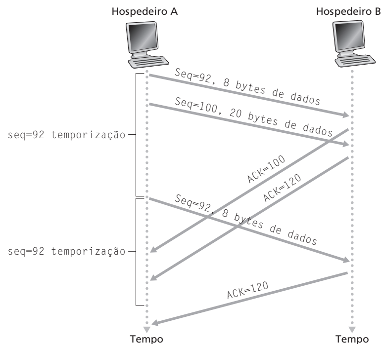
Figura 3.35 Segmento 100 não retransmitido
