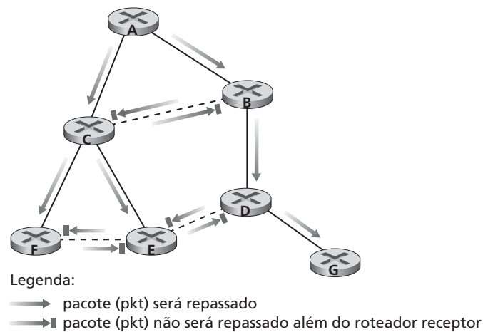
Figura 4.44 Repasse pelo caminho inverso
