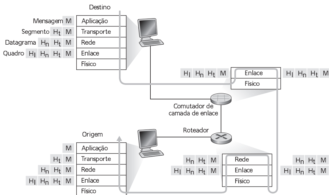
Figura 1.24 Hospedeiros, roteadores e comutadores de camada de enlace; cada um contém um conjunto diferente de camadas, refletindo suas diferenças em funcionalidade
