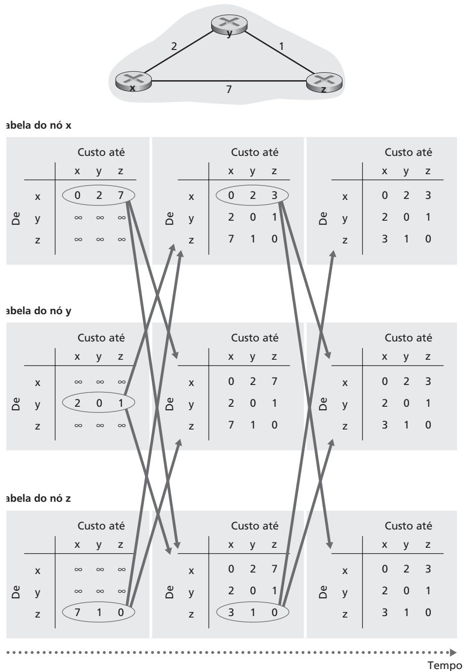
Figura 4.30 Algoritmo de vetor de distâncias (DV)
