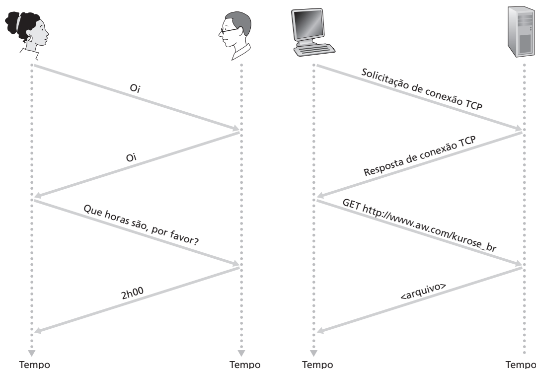
Figura 1.2 Um protocolo humano e um protocolo de rede de computadores
