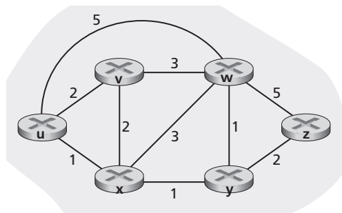
Figura 4.27 Modelo abstrato de grafo de uma rede de computadores
