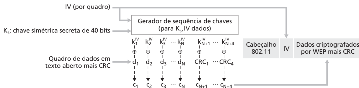
Figura 8.31 Protocolo 802.11 WEP
