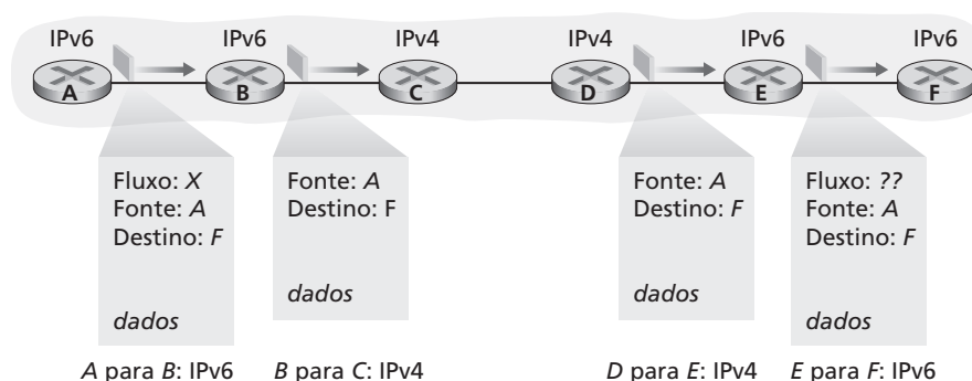
Figura 4.25 Abordagem de pilha dupla
