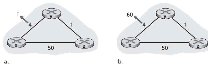
Figura 4.31 Mudanças no custo do enlace
