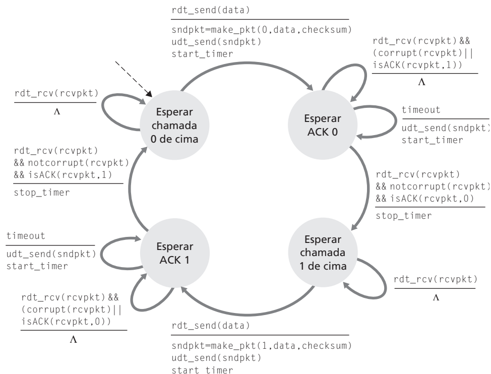
Figura 3.15 rdt3.0 remetente
