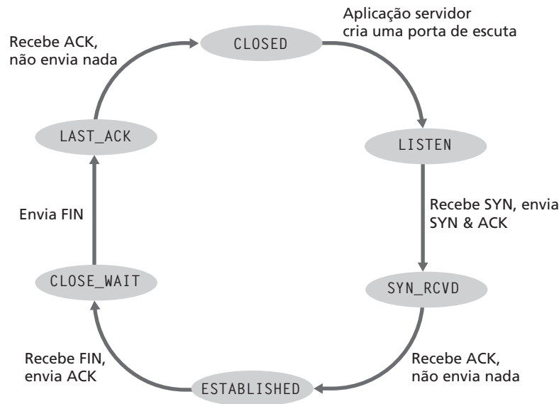
Figura 3.42 Uma sequência típica de estados do TCP visitados por um TCP do lado do servidor
