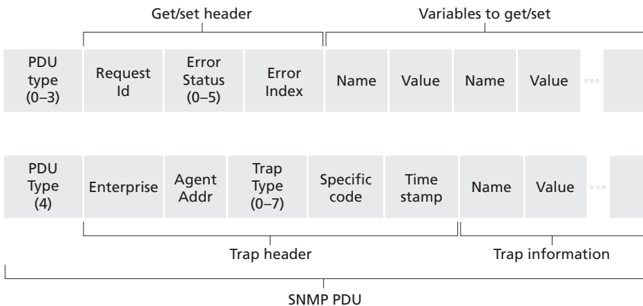
Figura 9.4 Formato da SNMP-PDU
