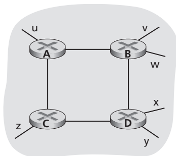
Figura 4.34 Número de saltos do roteador de origem, A, até várias sub-redes
