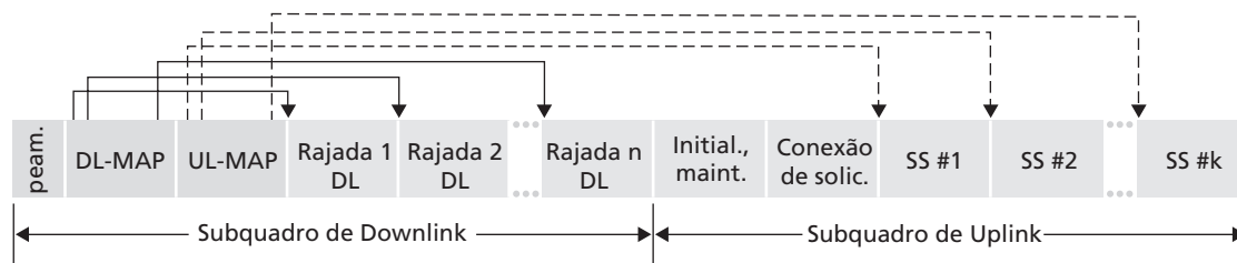
Figura 6.17 Estrutura de quadro 802.16 TDM
