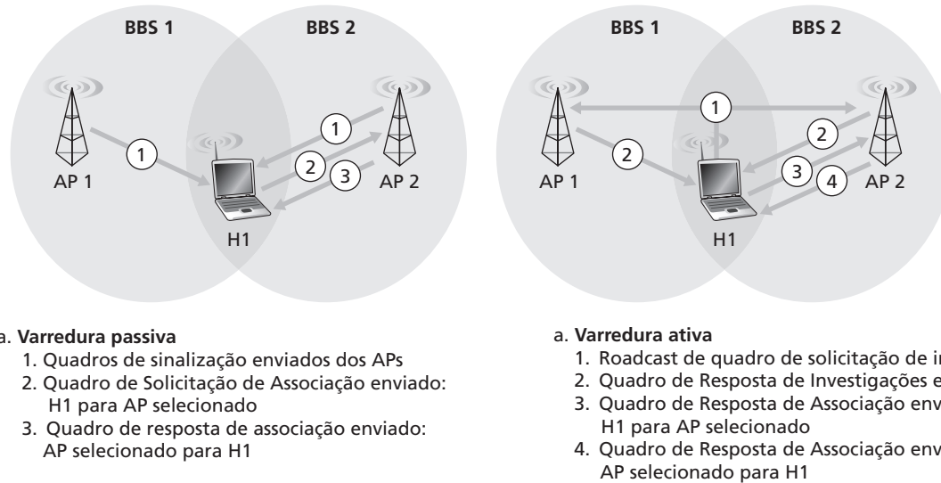
Figura 6.9 Varredura passiva e ativa para pontos de acesso
