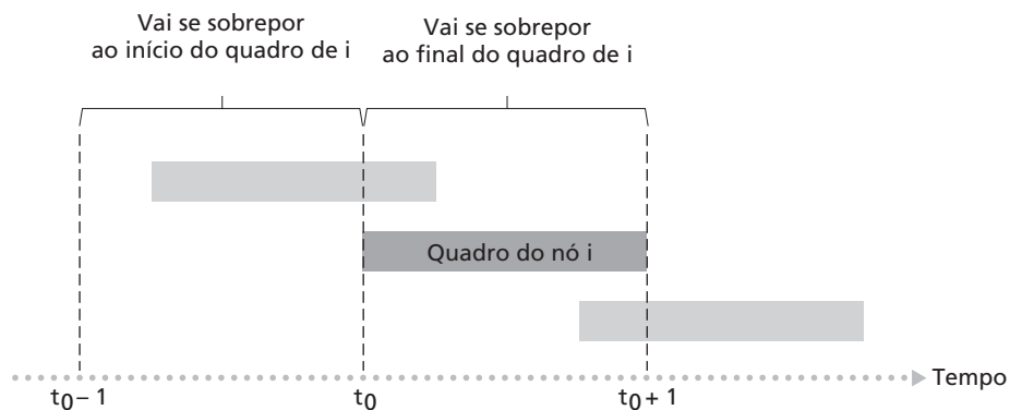
Figura 5.12 Transmissões interferentes no Aloha puro
