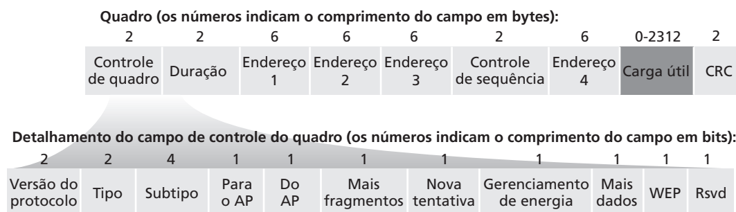
Figura 6.13 O quadro 802.11
