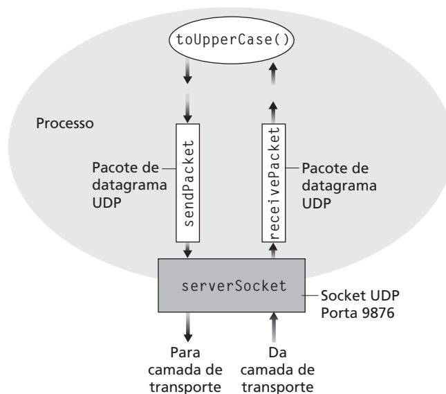
Figura 2.34 UDPServer não tem Cadeias; o socket aceita pacotes do processo e entrega pacotes ao processo
