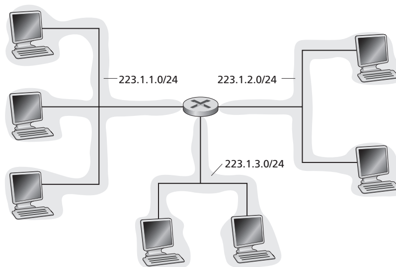
Figura 4.16 Endereços de sub-redes
