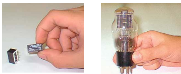
Figura 8. Relé e Válvula
