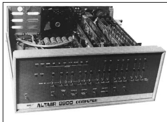
Figura 16. Altair
