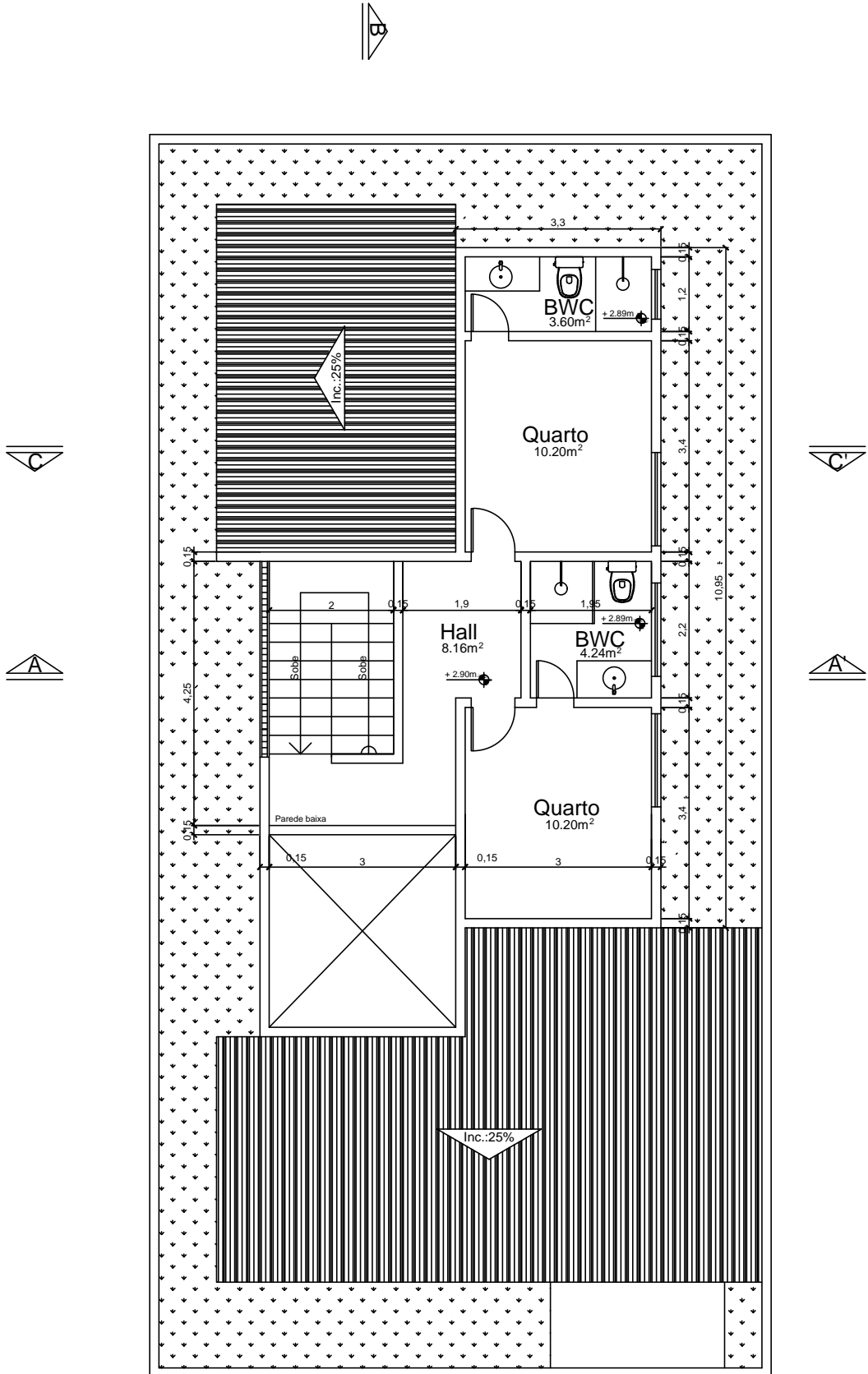
Planta pavimento superior
