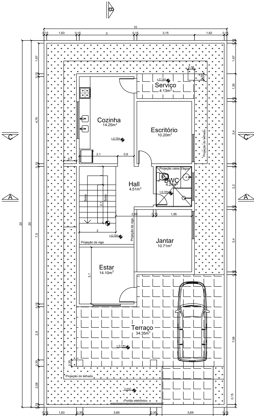
Planta pavimento térreo
