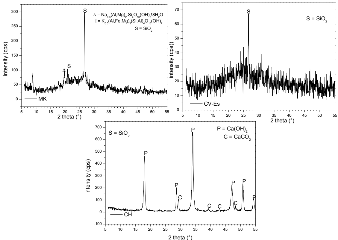
Fig 1. DRX da cinza volante (CV-Es), metacaulino (MK) e cal hidratada (CH)
