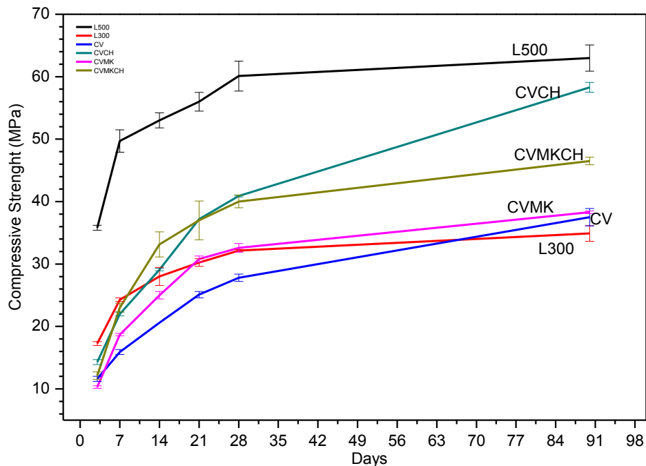
Fig. 6. Evolução das resistências à compressão com a idade
