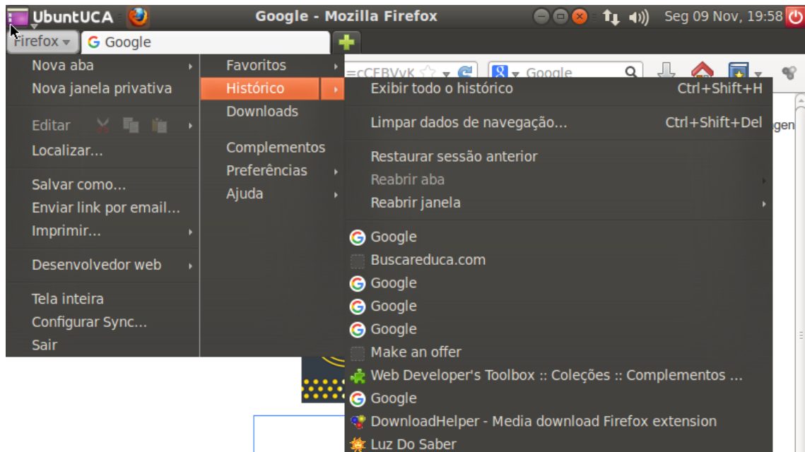
Figura 3.1.2.9 – Histórico.
