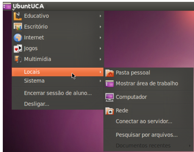
Figura 23. Menu Locais.
