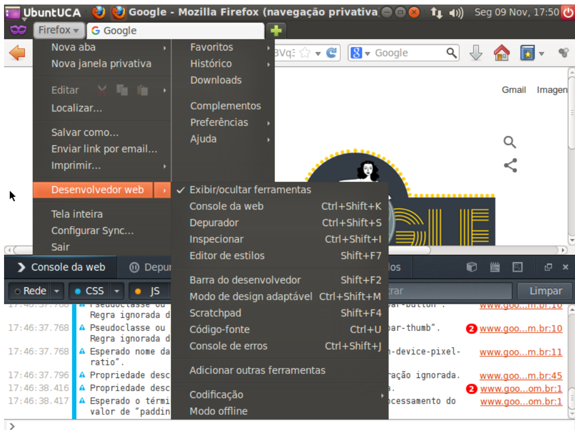
Figura 3.1.2.5 – Desenvolvedor web.
