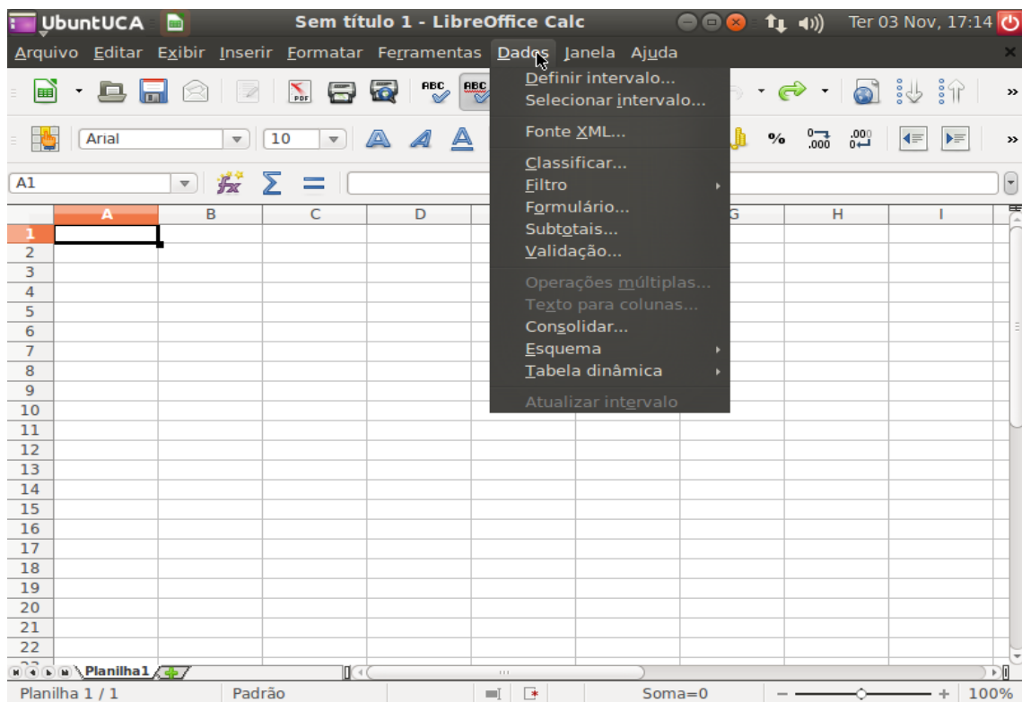
Figura 66 - Menu dados
