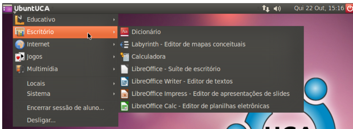
Figura 15. Menu Escritório.
