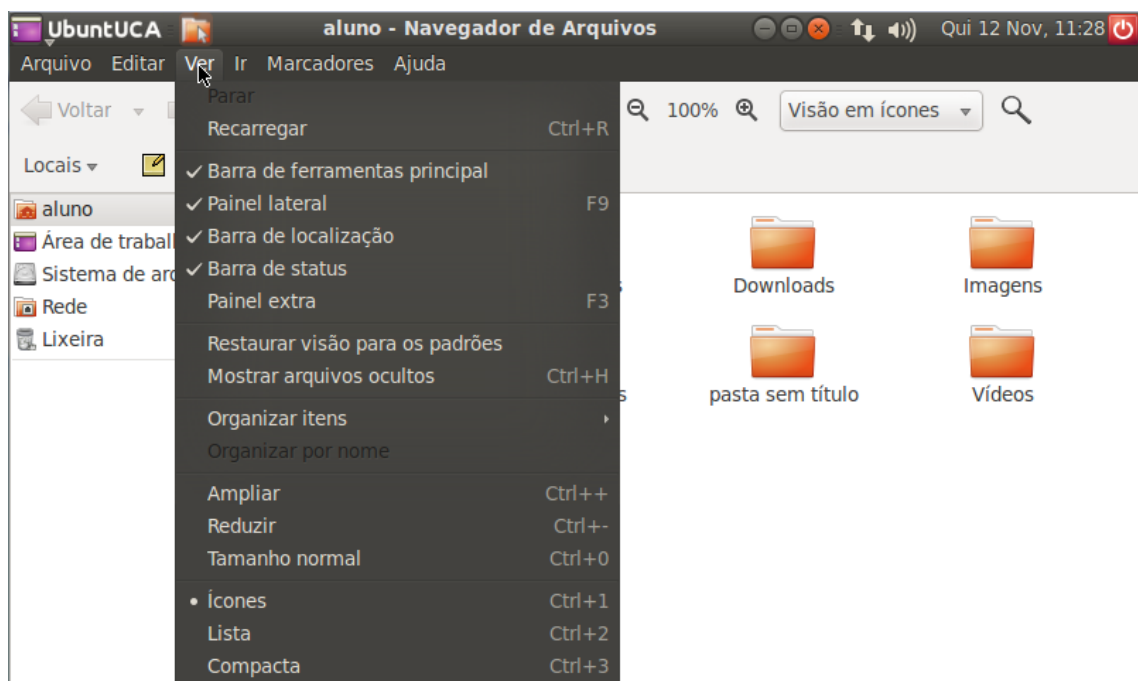
Figura 52. Meu Ver.
