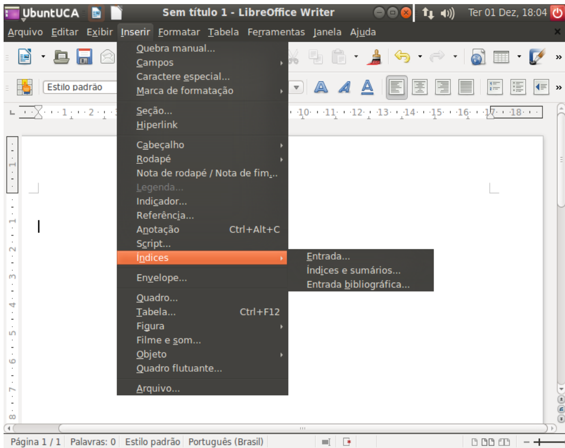
Figura 39: Índices
