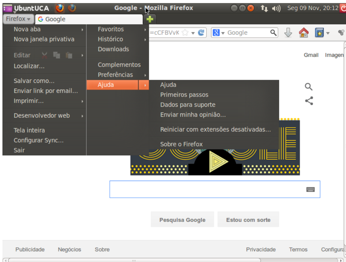
Figura 3.1.2.12 – Ajuda.
