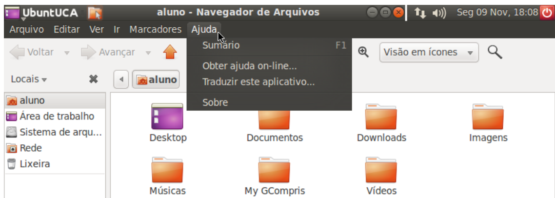
Figura 61. Menu Ajuda.
