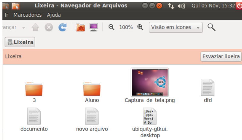
Figura 36. Esvaziar lixeira
