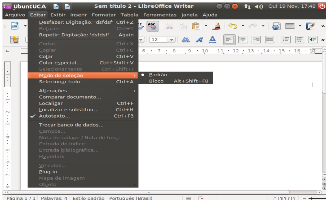
Figura 27: Modo seleção
