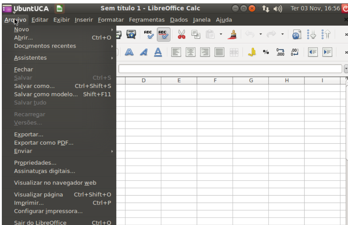
Figura 45 - Menu arquivo
