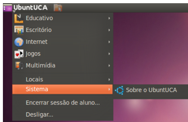
Figura 24. Menu Sistema.
