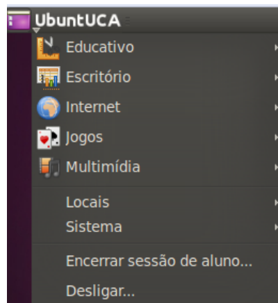
Figura 05. Menu UbuntuUCA
