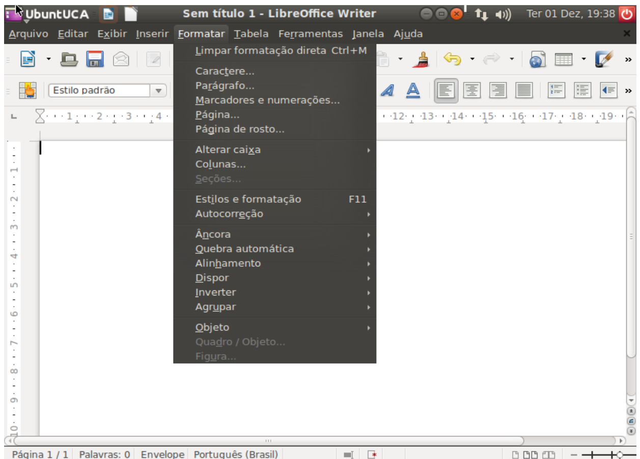
Figura 41: Limpar formatação
