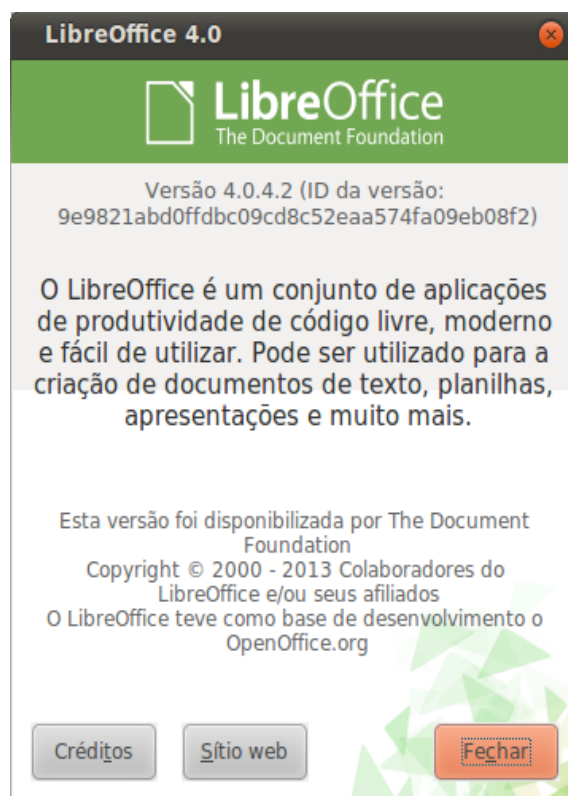
Figura 47: LibreOffice
