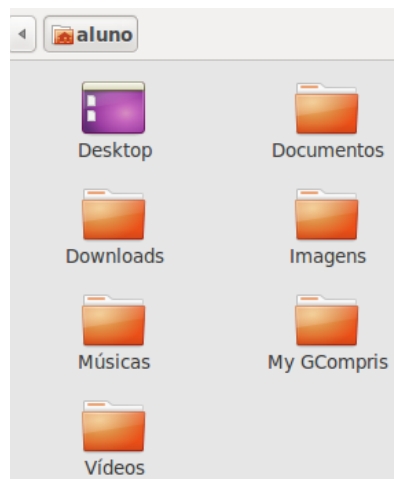
Figura 57. Painel extra.
