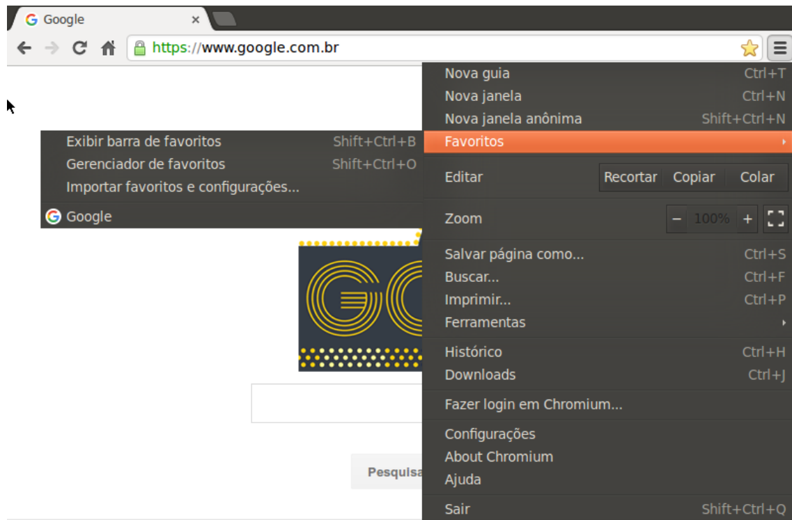
Figura 3.1.8 – Favoritos.
