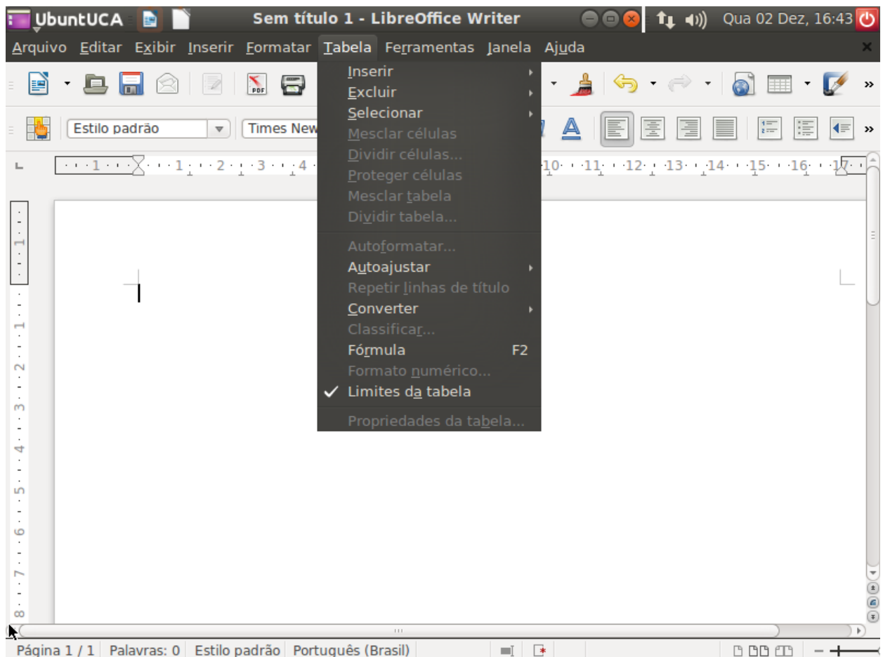
Figura 43: Tabela
