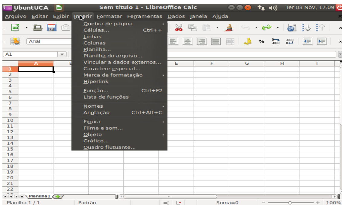
Figura 53 - Menu inserir
