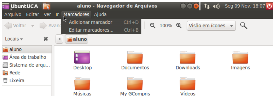
Figura 60. Menu Marcadores.
