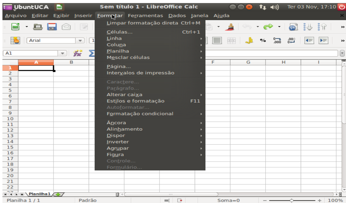
Figura 54 - Menu Formatar
