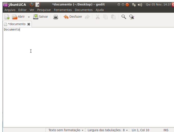
Figura 33. “Arquivo vazio”
