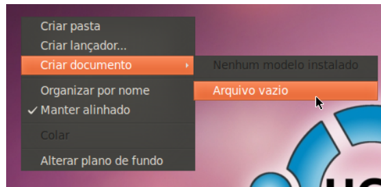
Figura 32. Criar documento.
