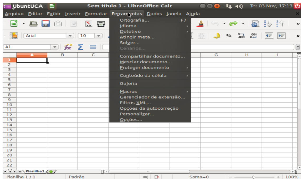
Figura 62 - Menu Ferramentas
