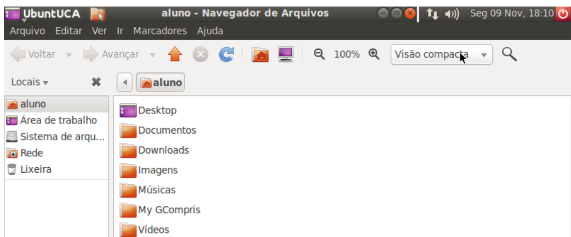
Figura 43. Visão compactada.
