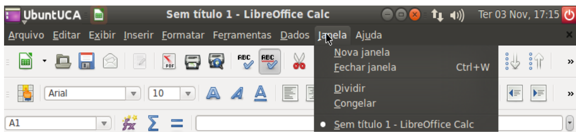
Figura 70 - Menu Janela
