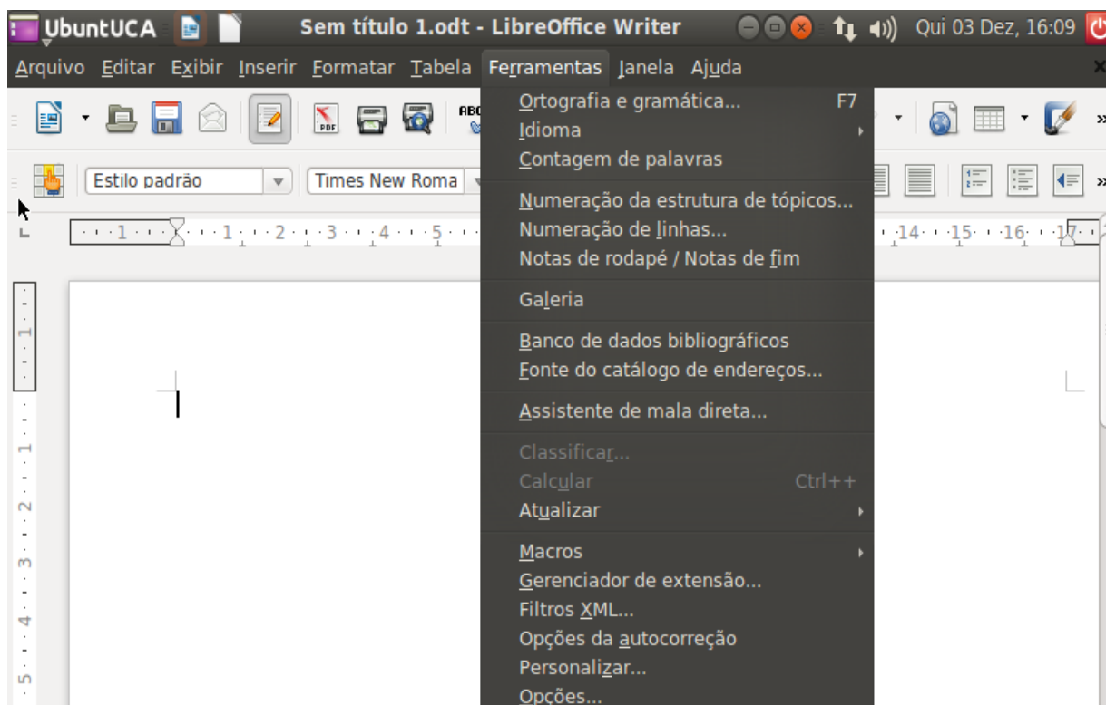
Figura 44: Ferramentas
