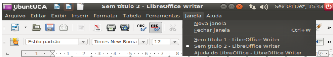
Figura 46: janela
