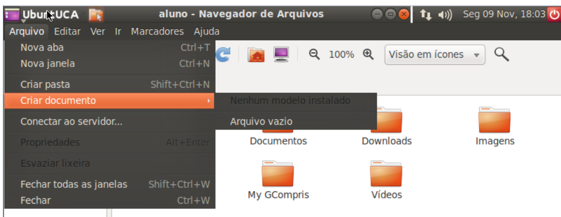
Figura 50. Menu Arquivo.
