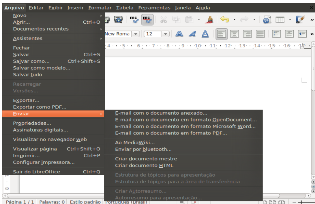
Figura 17: Aba Enviar
