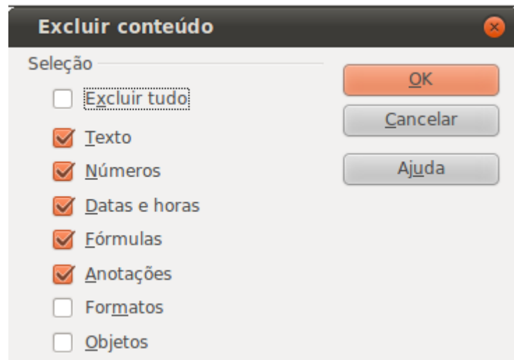
Figura 48 - Excluir conteúdo
