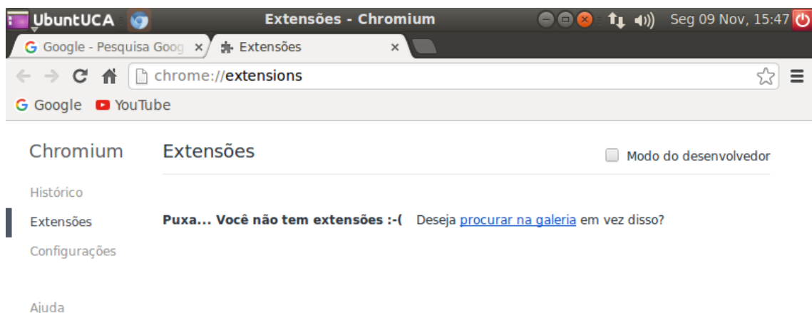
Figura 3.1.15 – Extensões.
