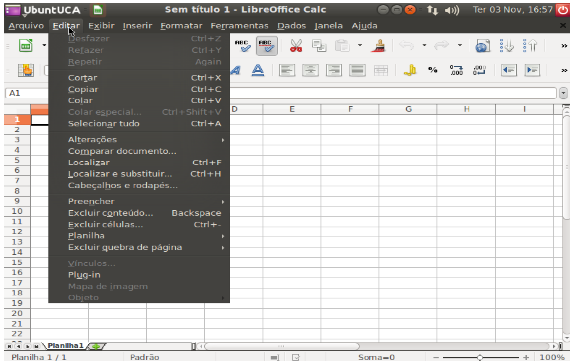
Figura 46 - Menu editar
