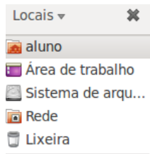
Figura 54. Painel lateral.
