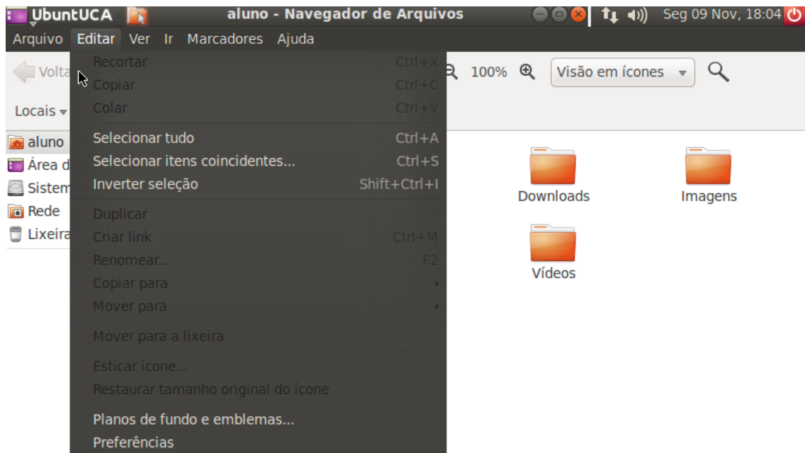
Figura 51. Menu Editar.
