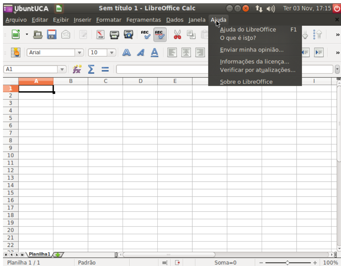
Figura 71 - Menu Ajuda
