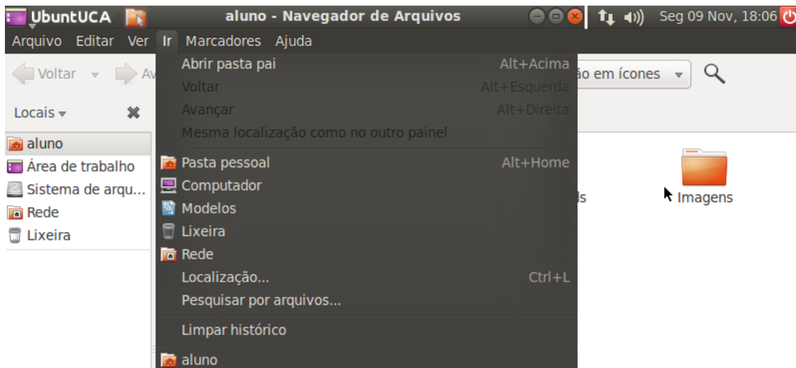
Figura 59. Menu Ir.
