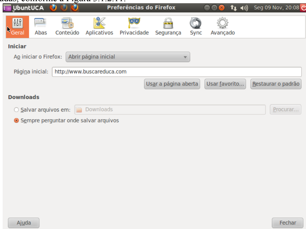
Figura 3.1.2.11 – Preferências.
