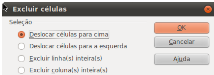
Figura 49 - Excluir células
