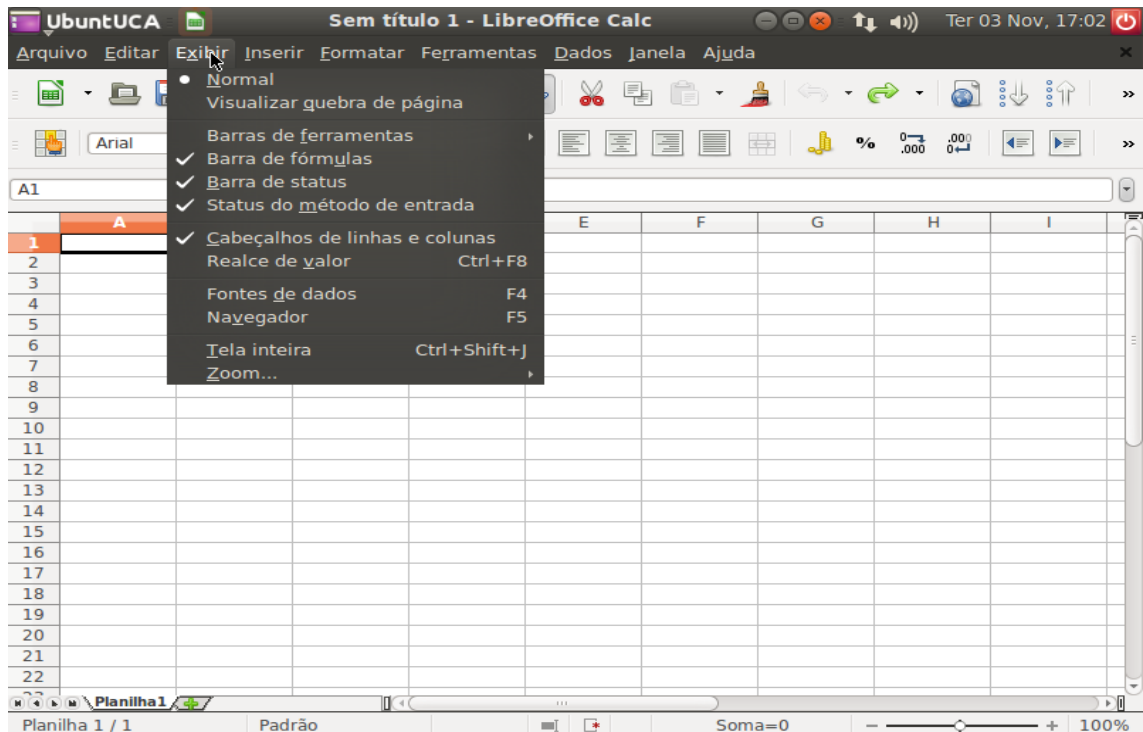
Figura 52 - Menu exibir
