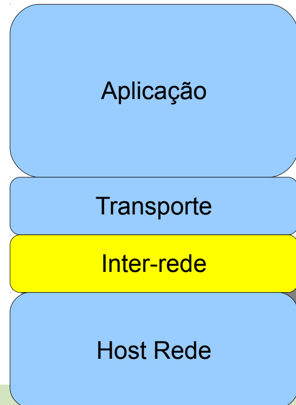
Modelo TCP/IP
