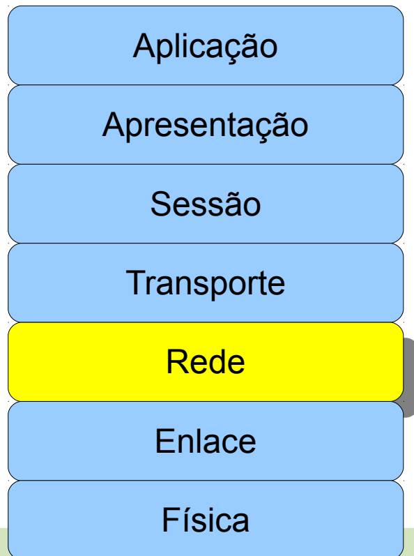
Modelo OSI
